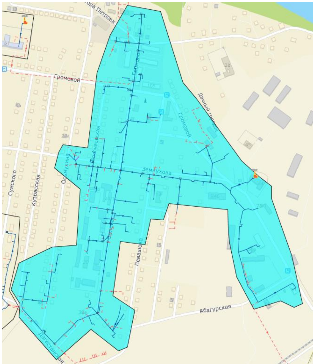
Рисунок 1.16 – Зона действия котельной №1 п. Абагур-Лесной
